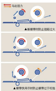
双碳带电机自动控制示意图 ▶
